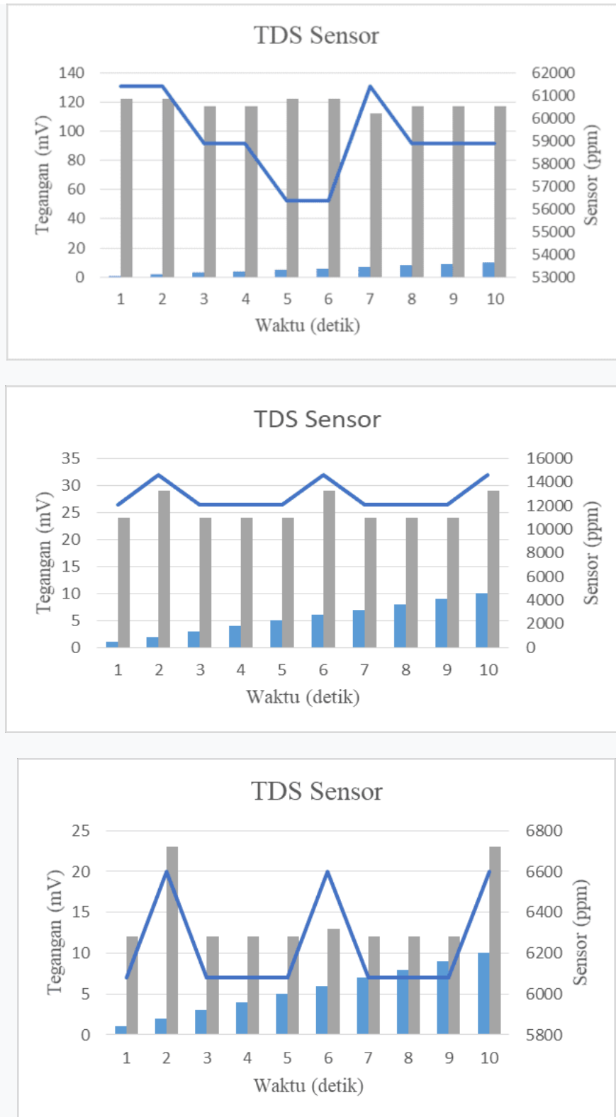
Gambar 11. Pengujian Sensor TDS dengan Beberapa Aturan Nutrisi
