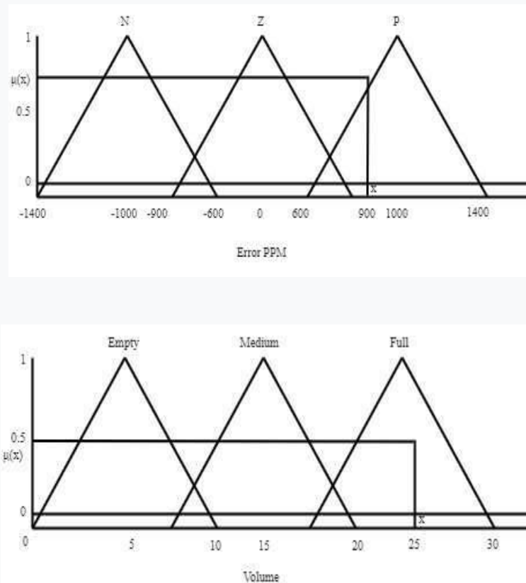
Gambar 5. Mambership Function pada Input Logika Fuzzy (A) Errorppm, (B) Volume
