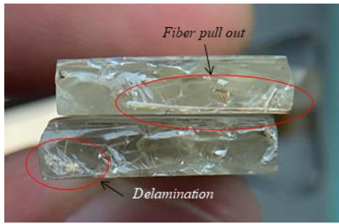
Gambar 2. Variasi Campuran (resin 75% : 25% serat)
