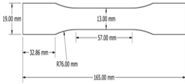
Gambar 1. ASTM D 638 tipe I
