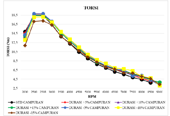
Gambar 3.4 Hasil Pengujian Torsi Berbahan Bakar Campuran
