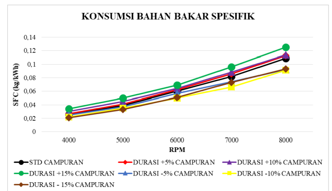
Gambar 3.6 Hasil Pengujian Konsumsi Bahan Bakar Spesifik Berbahan Bakar Campuran
