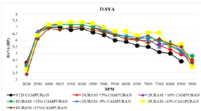
Gambar 3.2 Hasil Pengujian Daya Berbahan Bakar Campuran
