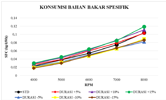
Gambar 3.5 Hasil Pengujian Konsumsi Bahan Bakar Spesifik Berbahan Bakar Pertamax
