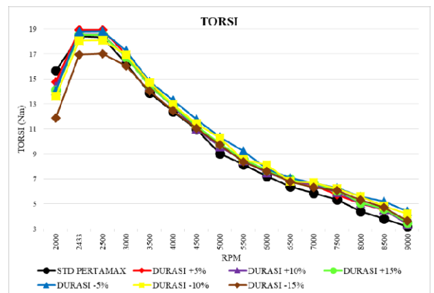
Gambar 3.3 Hasil Pengujian Torsi Berbahan Bakar Pertamax
