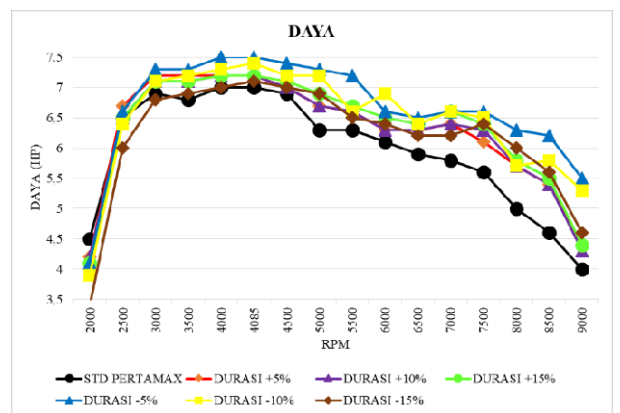
Gambar 3.1 Hasil Pengujian Daya Berbahan Bakar Pertamax
