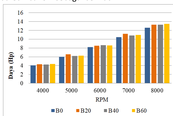
Gambar 3.2 Grafik perbandingan pengujian daya bahan bakar pertamax murni dan campuran bioetanol
